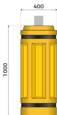
CP100
